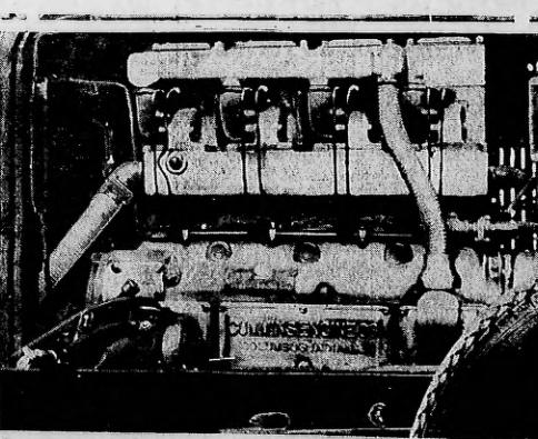
Este es el primer motor Diesel colocado en un automóvil y con el cual se realizaron las pruebas en Columbus (Indiana), lográndose establecer un promedio de 80 millas en una hora. La aplicación de este motor a los automóviles, revolucionará la industria automotriz
