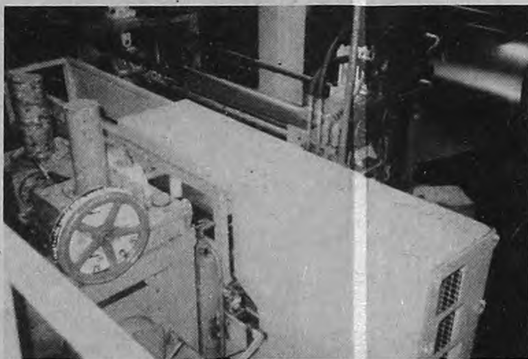
FOTOS DEL ELMES: EQUIPO LASER PARA MEDICION DE SUCIEDAD INSTALADOS POR EL CENTRO DE INVESTIGACIONES OPTICAS (CONICET) Y EL LABORATORIO DE ELECTRONICA CUANTICA DE LA FCEYN (UBA) EN LA EMPRESA SIDERAR.
