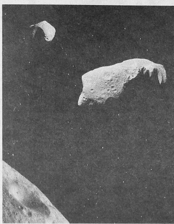
NORTEAMERICANA NEAR, A PRINCIPIOS DE 1999, SE PUSO EN SU ÓRBITA Y ALLÍ CONTINUA.
