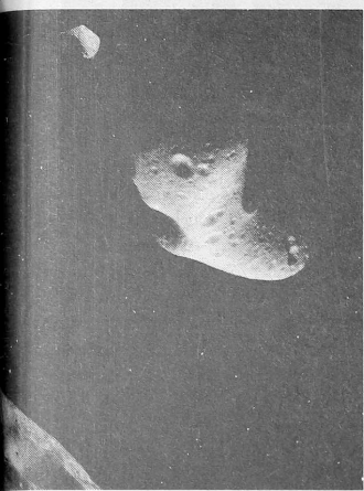
NORTEAMERICANA NEAR, A PRINCIPIOS DE 1999, SE PUSO EN SU ÓRBITA Y ALLÍ CONTINUA.
