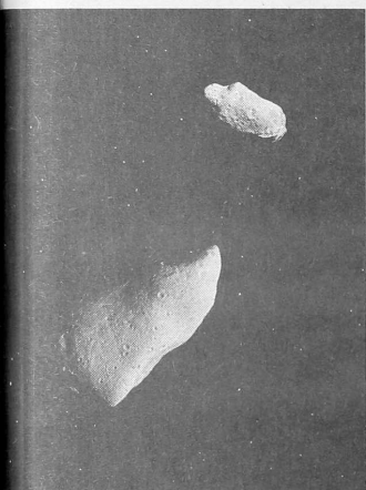
DOS ASTEROIDES IDA Y GASPARA
