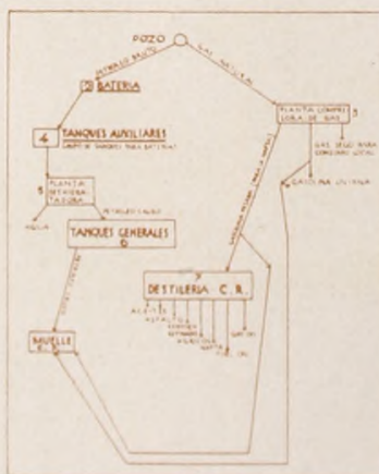
Esquema general de la elaboración del petróleo en Comodoro Rivadavia.
