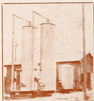
Vista parcial de la Planta Gasolina.
