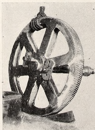
Engranaje en hierro fundido, diámetro 1.20 mts. so'dado en los talleres Gourinski, Buenos Aires, con
