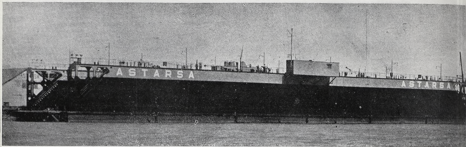
Dique Flotante ASTARSA. Construcción N° 95. — Construcción efectuada en gradas por secciones y unidas las mismas a flote. Posee las siguientes características: 108,20 mts. de eslora, 24,20 de manga y 10,40 de puntal con una capacidad portante de 2.800 Tn., 6 pontones y 2 cajones laterales en los cuales están instaladas sus maquinarias y taller de mantenimiento. Construido durante los años 1955/56 para el M. T. N.
