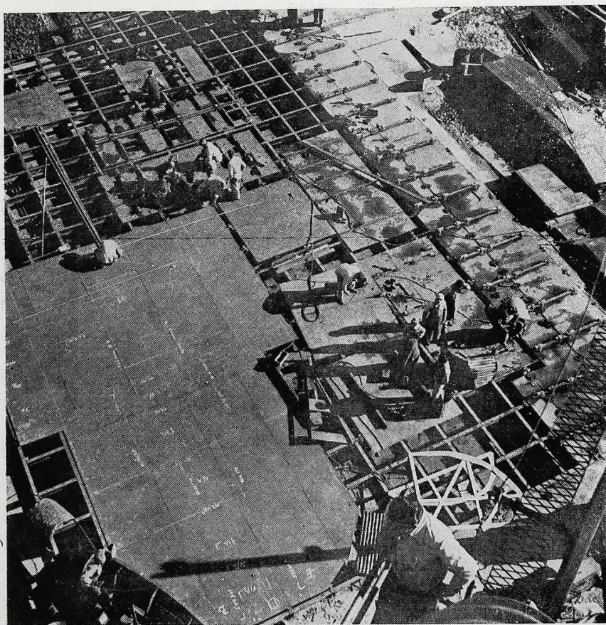
Plato de soldadura para grandes trozos.
