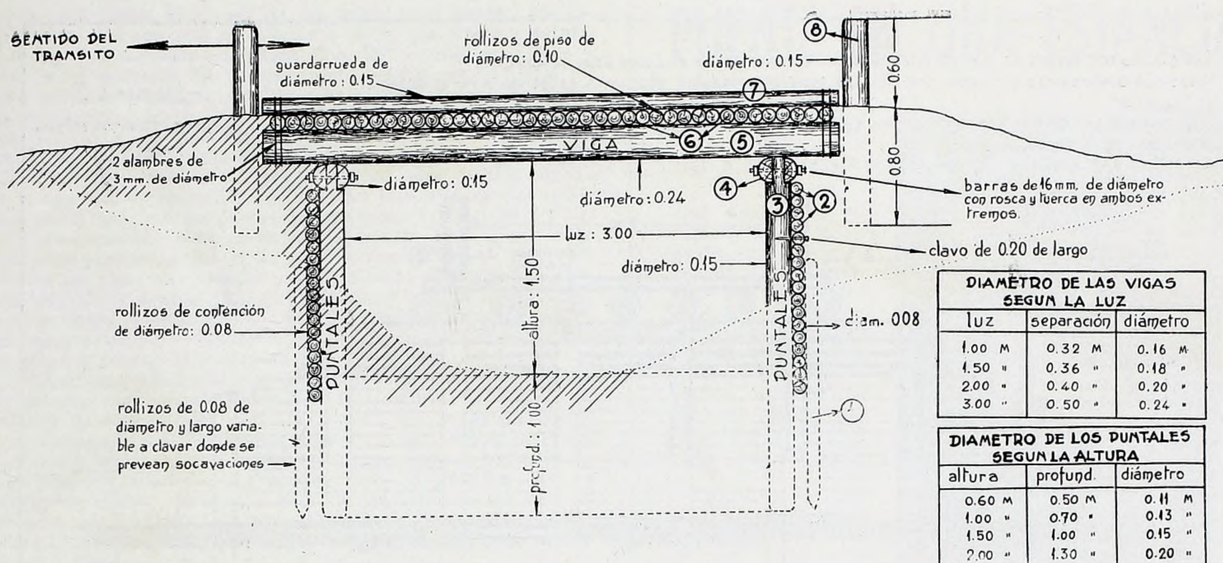
Figura 1 — Corte longitudinal — Escala: 1: 25
