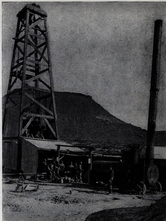
El histórico pozo N° 2 de la zona de Comodoro Rivadavia, que marcó la fluencia inicial de petróleo en la Patagonia el 13 de diciembre de 1907
