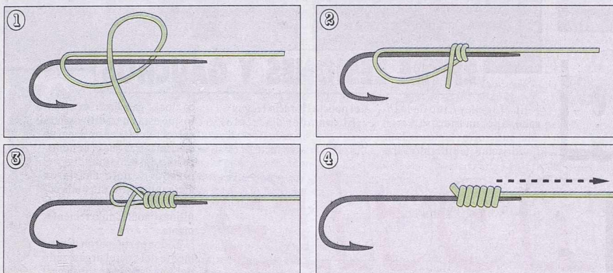
Nudo para anzuelo de paleta.
