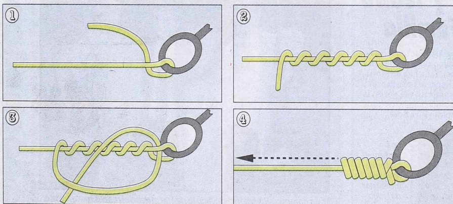
Nudo para mosquetones y esmerillones.
