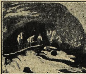
El agua en cavernas subterráneas Salida de agua de una caverna
