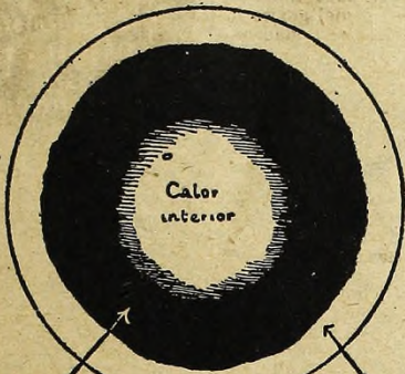
Corte de la tierra y el mar, en su estado actual
