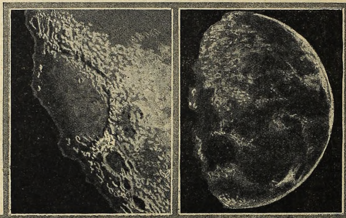
El llamado "mar de las Crisis"
