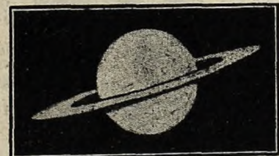
Saturno y sus anillos el 16 de julio de 1906
