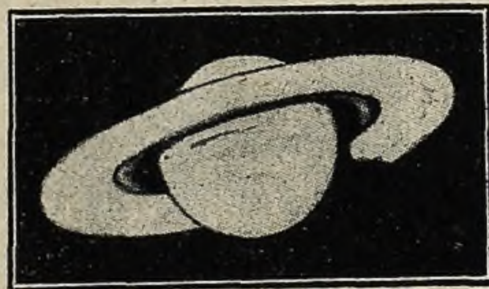
Saturno y sus anillos, según Trouvelot
