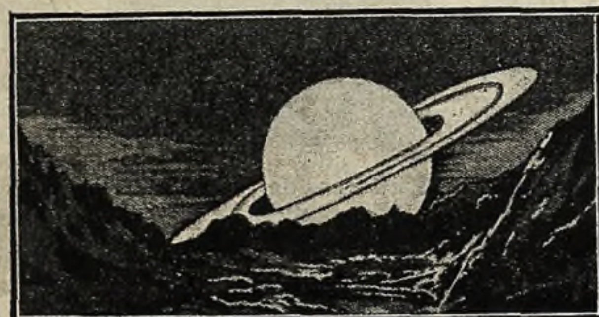
Orto de Saturno, desde su primer satélite
