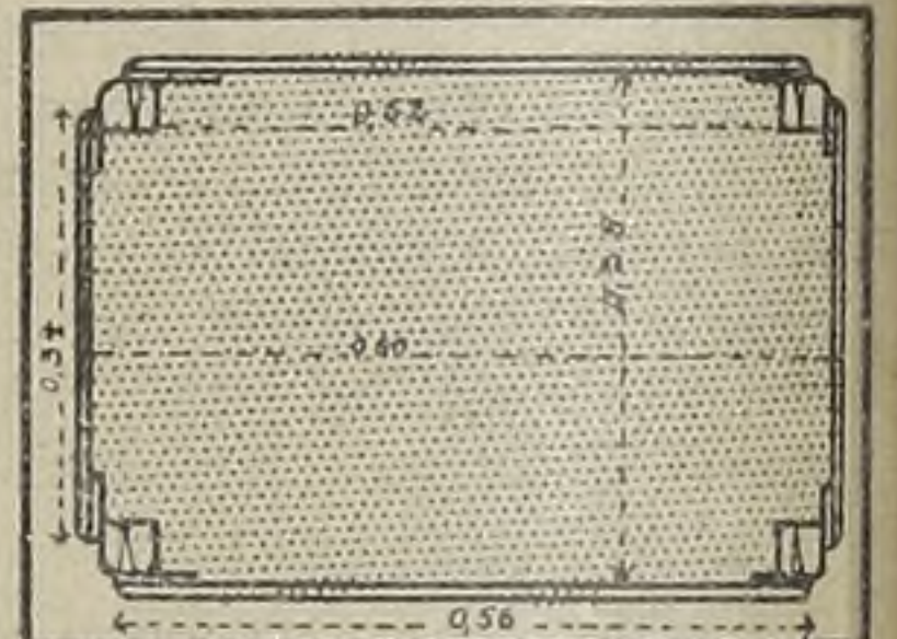
Plano y dimensiones de un entrepaño
