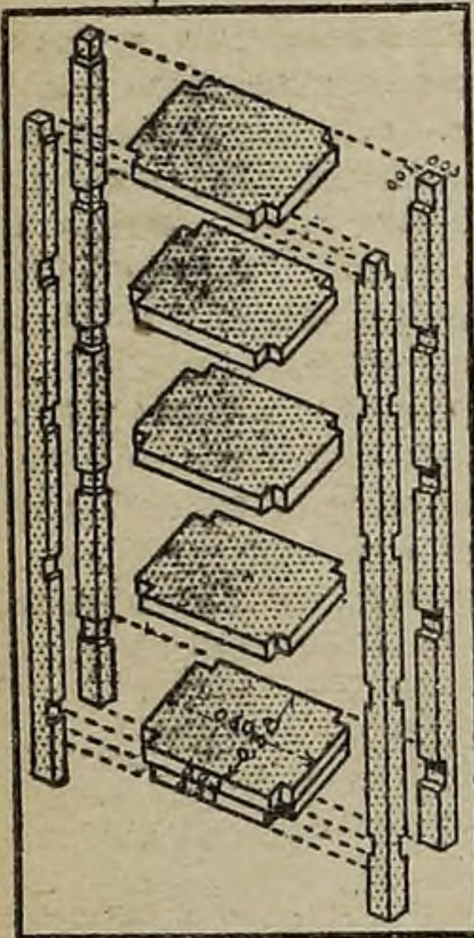
Los cinco tableros entallados en cada ángulo, se embuten en los montantes entallados, asimismo a la altura correspondiente
