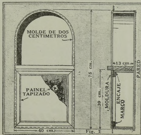
FRENTE Y CORTE SECCIONAL DEL NICHOPARA TELEFONO TERMINADO
